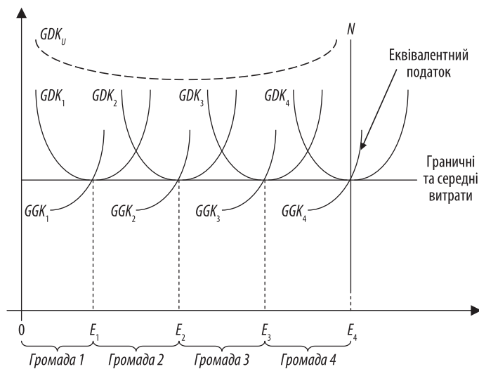
Модель Тьебу
