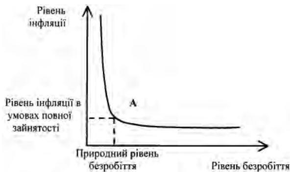
Крива Філіпса
