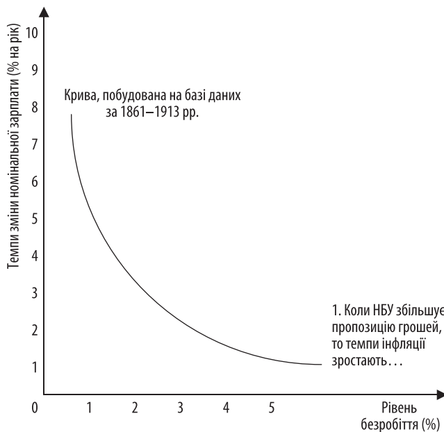
Крива Філіпса
